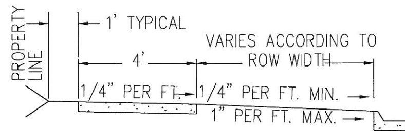
SECTION A-A
